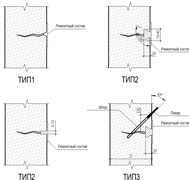
Рисунок 7.3 Схема ремонта трещин
