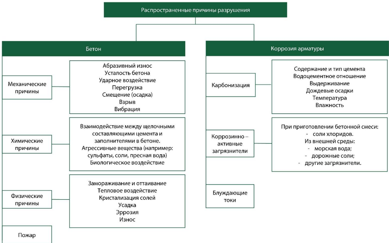
Рисунок Б.5 Наиболее вероятные причины проявления основных дефектов при эксплуатации железобетонных конструкций по ГОСТ 32016-2012
