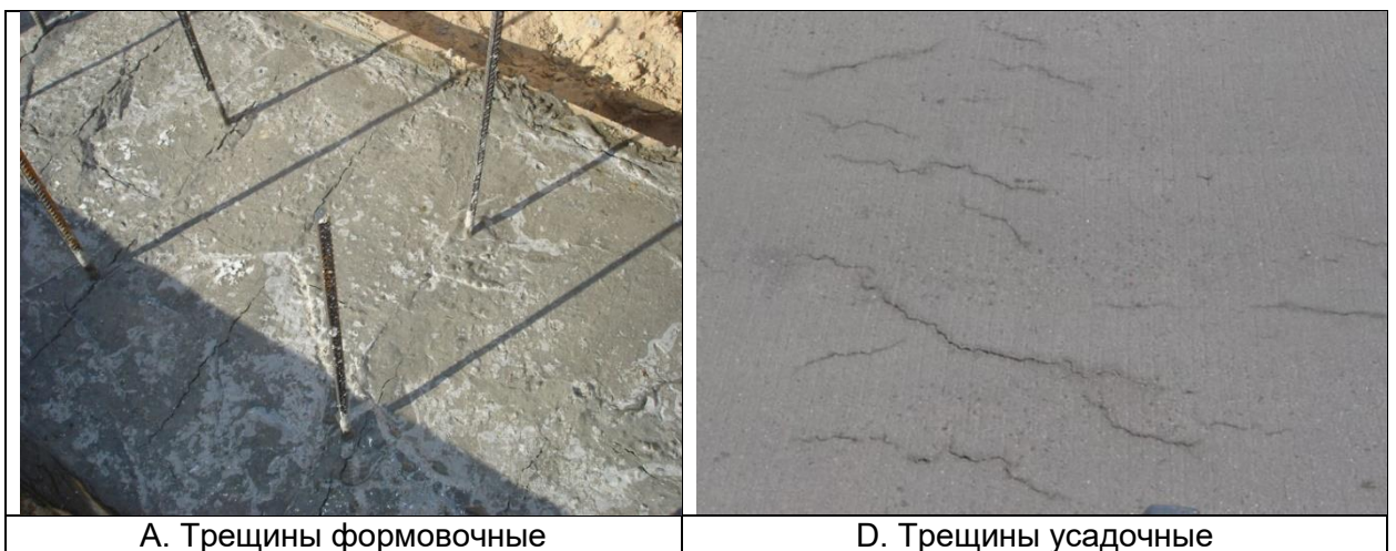
Рисунок Б.2 Характерные трещины в железобетонных конструкциях. Фотоизображения.
